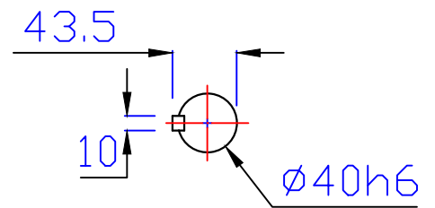
出力軸 Output Shaft
