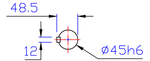
出力軸 Output Shaft
