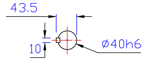
出力軸 Output Shaft
