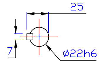
出力軸 Output Shaft
